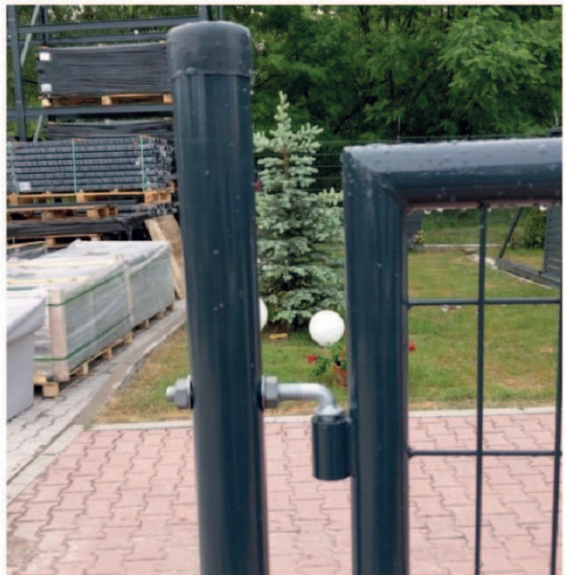
Zawiasy regulowane.
